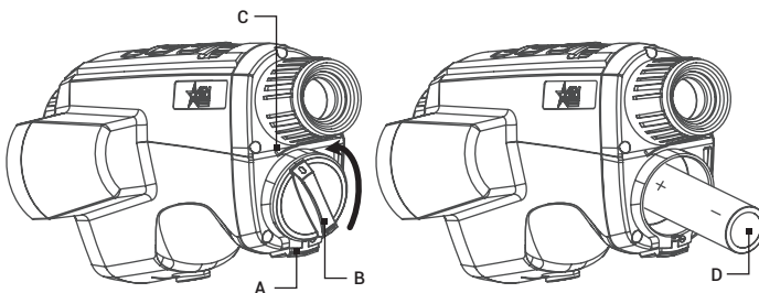
ABBILDUNG 2-1. EINLEGEN DER BATTERIEN
