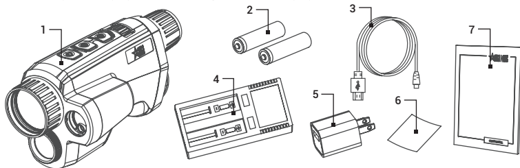
ABBILDUNG 1-2. STANDARDKOMPONENTEN
