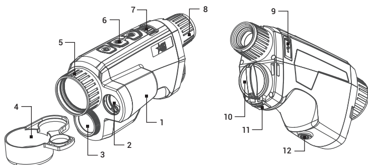
ABBILDUNG 1-1. HAUPTTEILE
