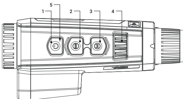
ABBILDUNG 2-2. STEUERTASTEN
